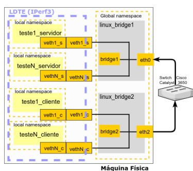
Fig. 3. Loopback lógico para homologação da máquina hospedeira da VALIDA.
